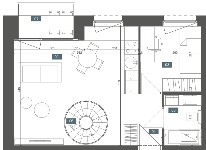
POZIOM I
