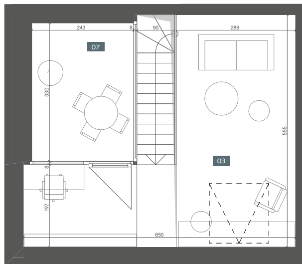
POZIOM II
